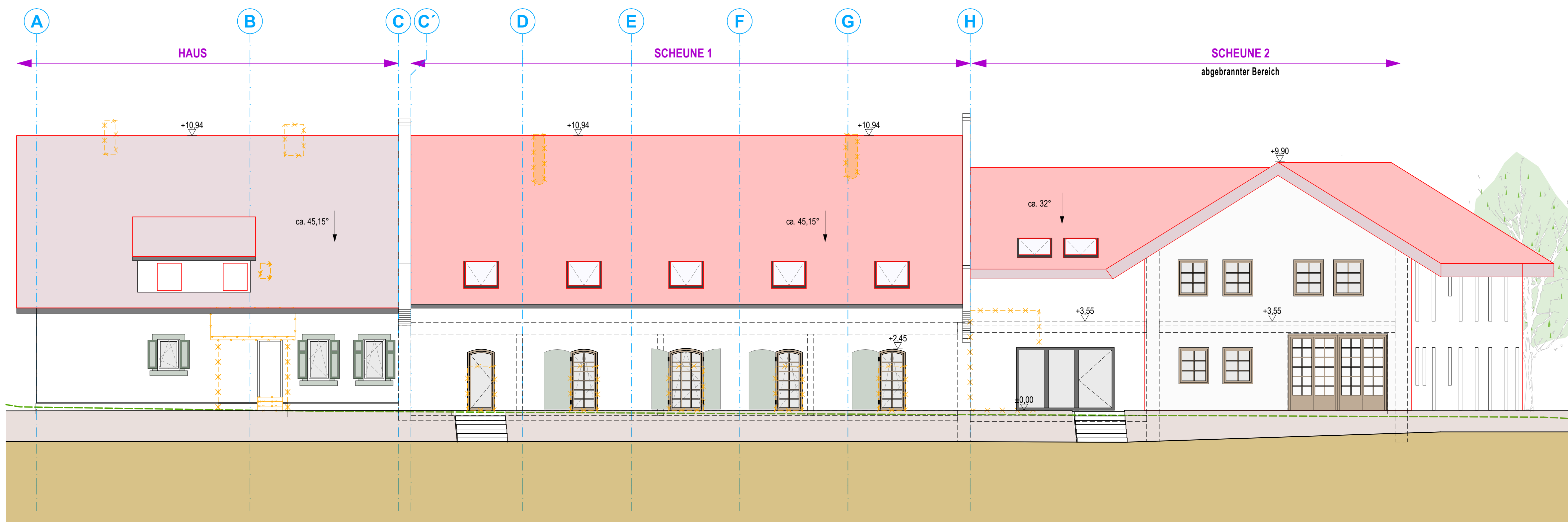
Ansicht Ost
