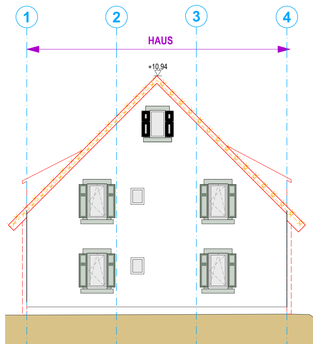
Ansicht Süd
