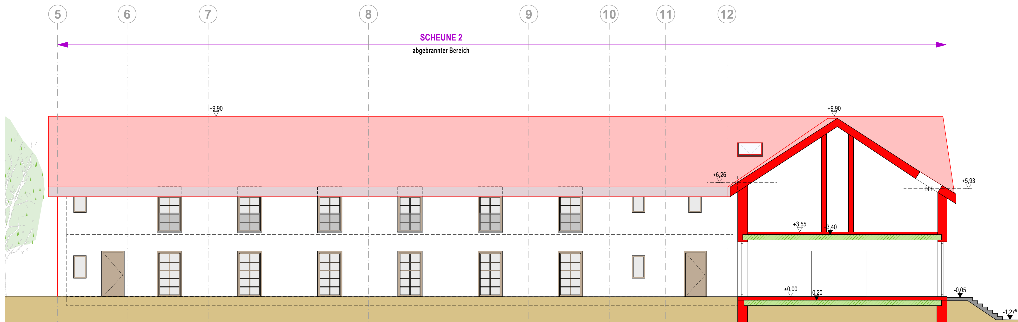
Ansicht Süd
