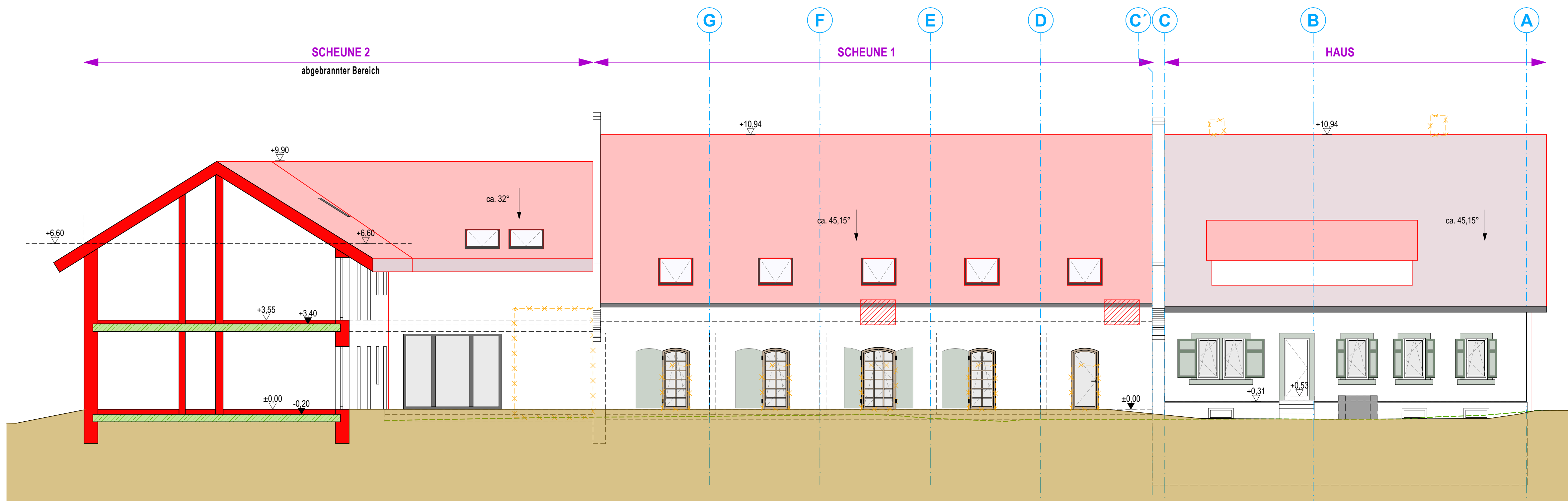
Ansicht West
